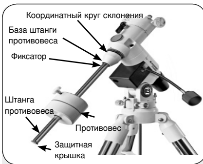
Рис. 6а: Монтровка, штанга противовеса и противовес в сборе (EXOS-2)
