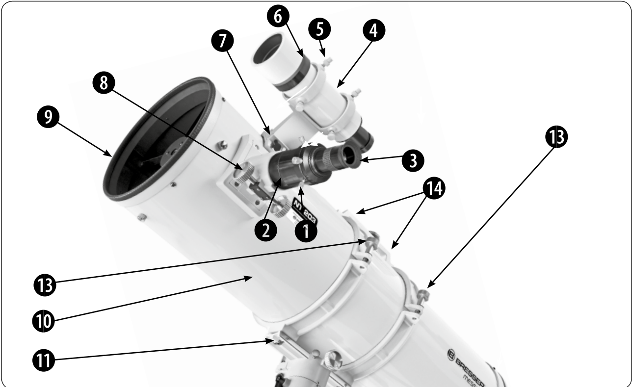
Рис. 1а. Телескопы серии Messier комплектуются искателем. Оптический узел в сборе (изображен рефлектор Ньютона)
