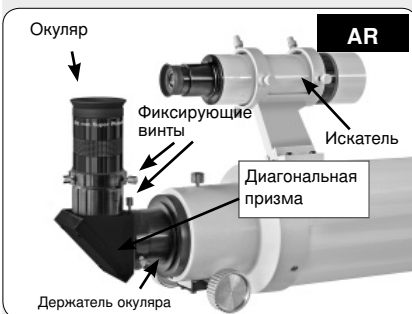
Рис. 10b: Вставьте окуляр в диагональную призму и затяните фиксирующие винты
